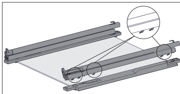
Fig. 51 Skleněná deska s koležnicemi a přídržnými díly
